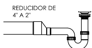
REDUCIDOR DE 4" A 2" DETALLE DE SIFON DE PILA 6 CODOS DE 2"
