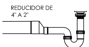
REDUCIDOR DE 4" A 2" DETALLE DE SIFON DE DUCHA 6 CODOS DE 2"
